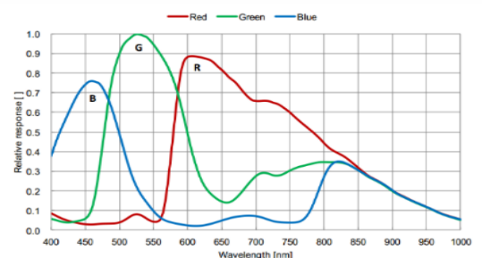
MV-CA023-10UC 量子效率
